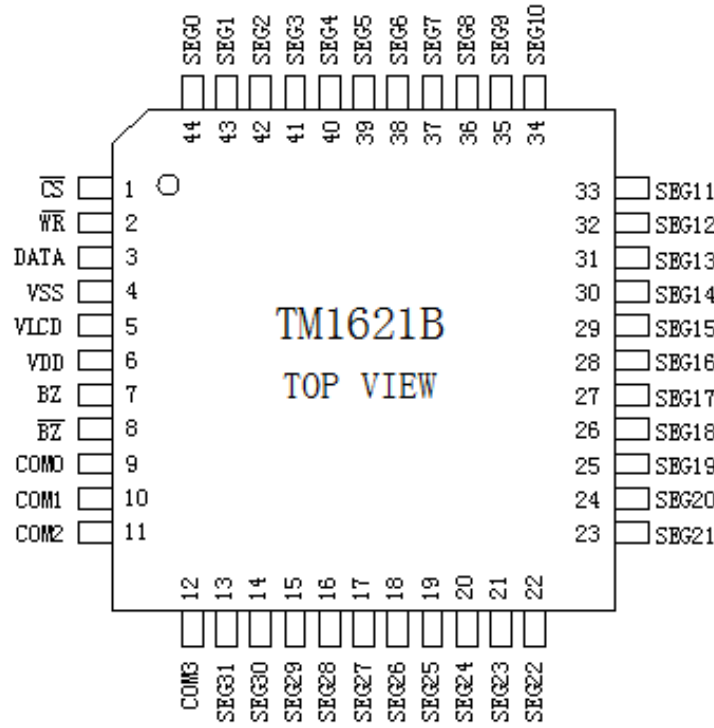
TM1621B_LQFP44
