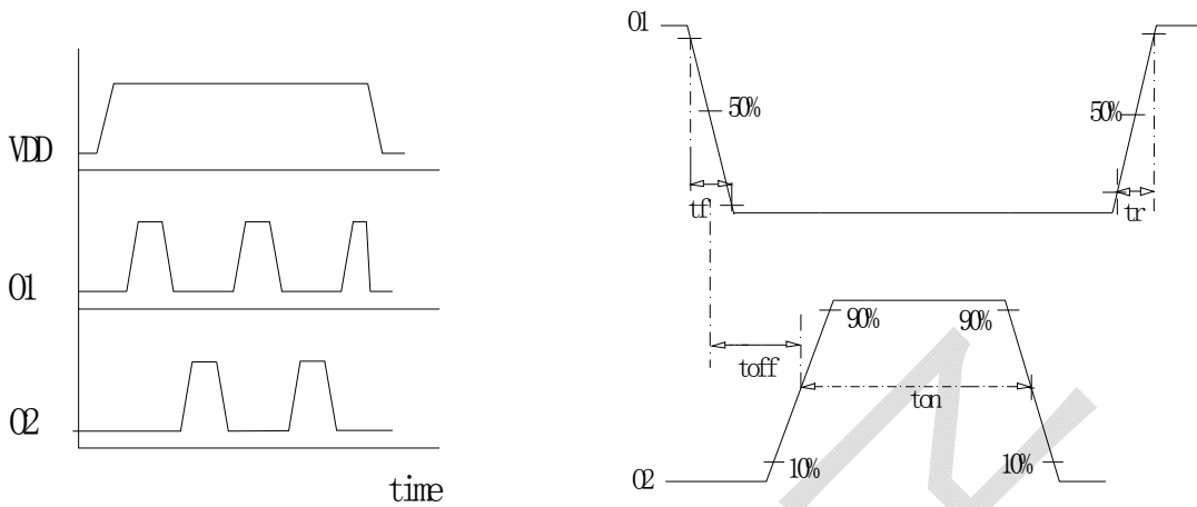
图2 输出波形图
